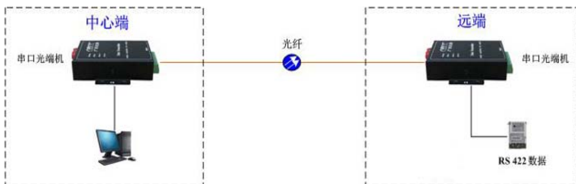
光纤点对点组网
